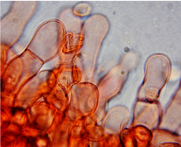
Cellules de la marge
