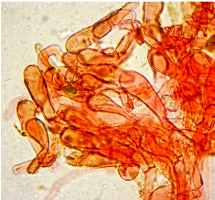
Caulocystides du sommet du pied
